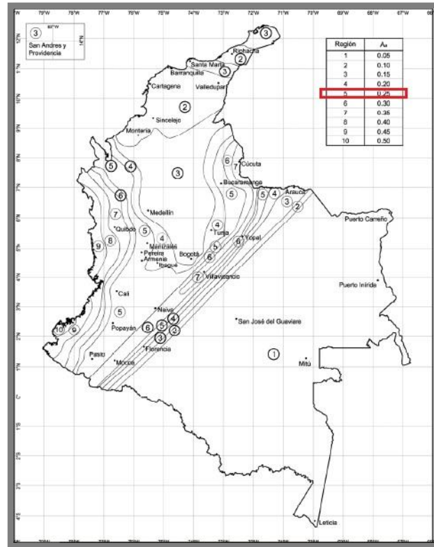
Figura 32. Gráfica de que representa la amenaza sísmica en Colombia, dividiendo el territorio en zonas de baja, intermedia y alta sismicidad. Nótese que el municipio de La Merced se encuentra en la zona 5 para la cual el A_a=0.25 . Fuente: Reglamento Colombiano de Construcción Sismo Resistente (2010).
