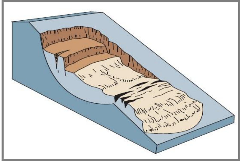
Figura 21. Esquema de un deslizamiento de tipo rotacional. Fuente: The Landslide Handbook (USGS, 2008).
