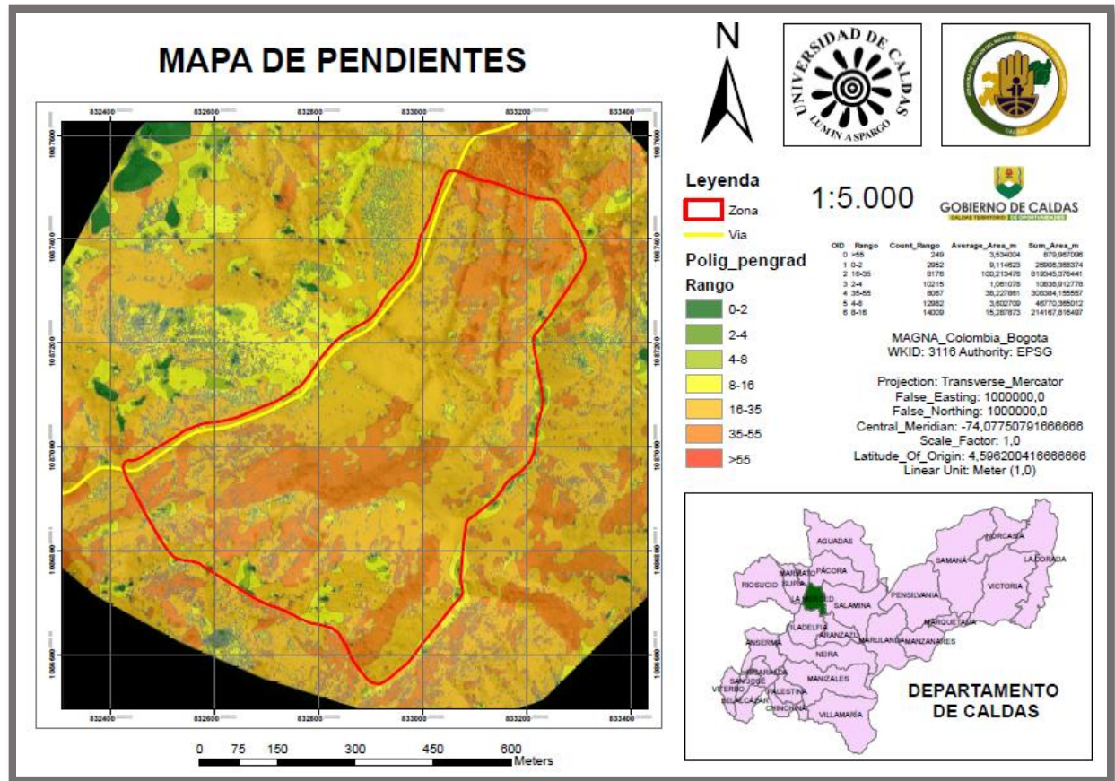
Figura 42. Mapa de pendientes para la zona de estudio. Nótese que la mayoría de la zona de estudio se encuentra entre los rangos de pendiente de 16°-35° clasificado como un terreno abrupto y 35°-55° como un terreno muy abrupto según el SGC. Fuente propia.
