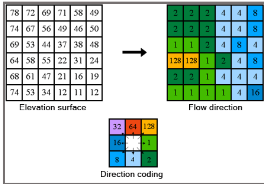
Figura 43. Modelo de flujo de ocho direcciones de salida válidas que se relacionan con las ocho celdas adyacentes hacia donde puede ir el flujo. Fuente: http://desktop.arcgis.com .
